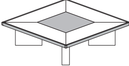
CX1624A L160 P160 H75 CX1625A L180 P180 H75 CX1630A L210 P210 H75
